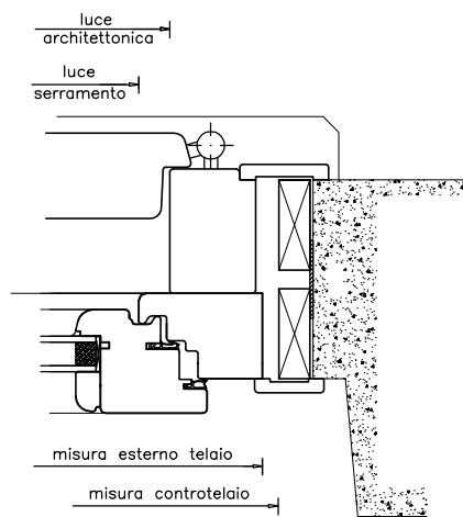
MONOBLOCCO
