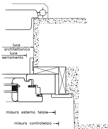
TRADIZIONALE CON RISVOLTO IN LEGNO
