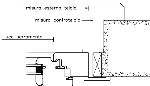
CONTROTELAIO IN LUCE
