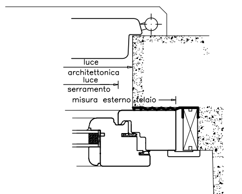
TRADIZIONALE CON RISVOLTO IN ALLUMINIO
