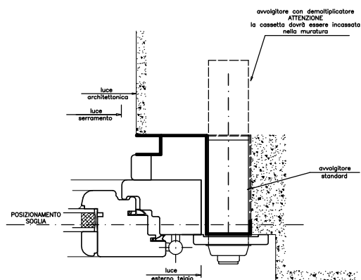
UNIBLOC A CINGHIA
